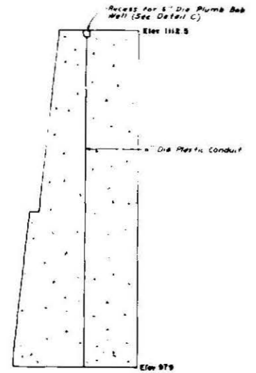
SECTION B-B SCALE: 1/8" = 1'-0"
