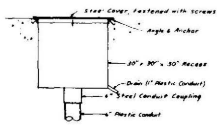
DETAIL C SCALE: 1/2" = 1'-0"
