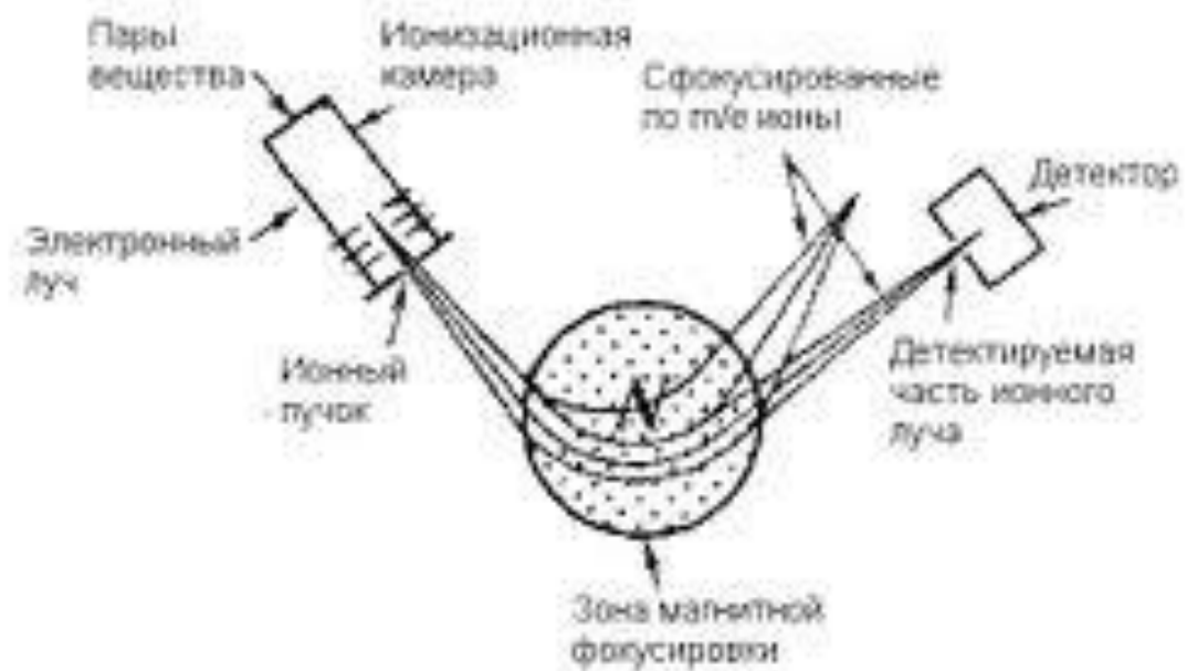
Схема устройства и работы масс-спектрометра
