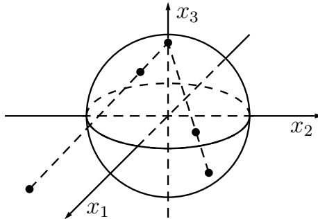
Рис. 1. Сфера Римана
