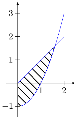
FIGURE 20.18: La région A de l'exemple 20.189. LabelFigExampleIntegration
