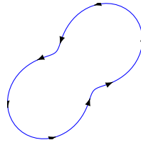
FIGURE 24.1: Un contour avec son orientation. LabelFigVDFMooHMmFZr
