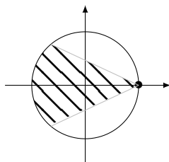
FIGURE 20.4: La zone dans laquelle peut être le chemin qui va vers z \rightarrow 1
