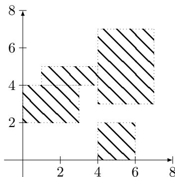
FIGURE 20.15: Un ensemble pavable. LabelFigPolirettangolo
