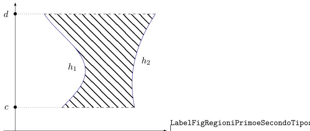
(b) Une region du deuxième type
