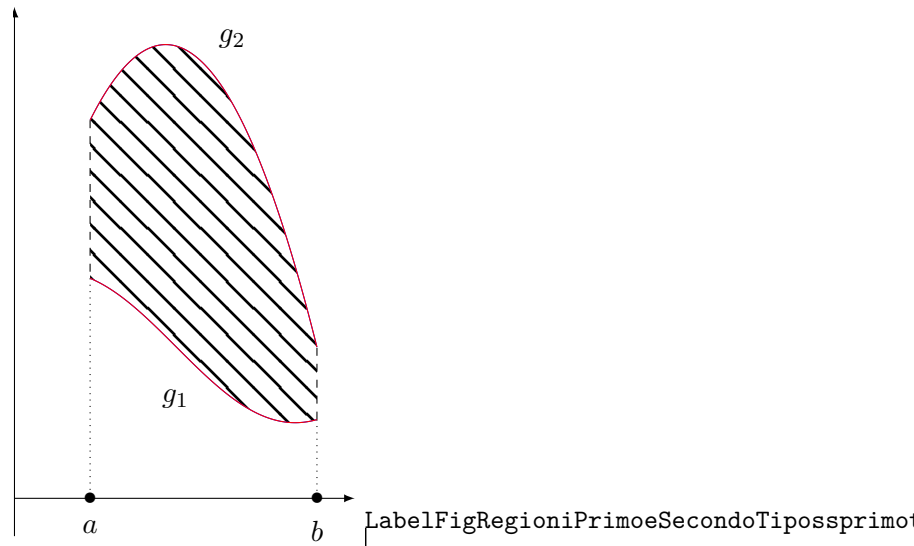
(a) Une region du premier type
