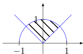
FIGURE 20.20: Il faut voir ça en trois dimensions. LabelFigCornetGlace
