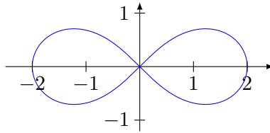
FIGURE 20.10: Intégrer sur des domaines plus complexes. Label: FigPONXooXYjEot
