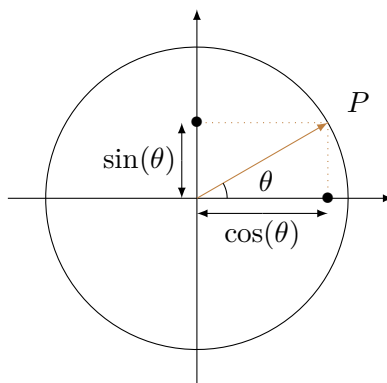
FIGURE 18.6: Le cercle trigonométrique. LabelFigCercleTrigono
