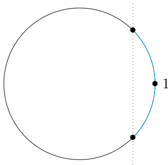
FIGURE 27.1: Un voisinage de 1 dans S^1 . LabelFigJQQVoolPTsYPZK
