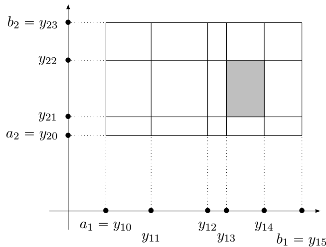
FIGURE 20.16: Une cellule d'une subdivision d'un pavé de \mathbb{R}^2 . La cellule grisée est R_{(k_1, k_2)} .
