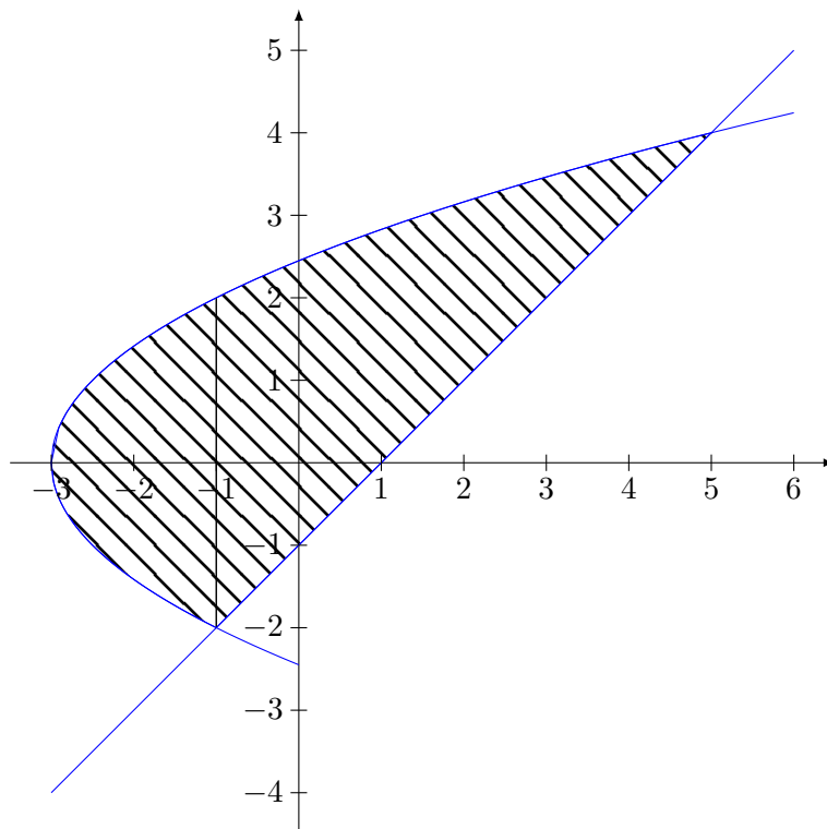
FIGURE 20.19: La région D de l'exemple 20.192. Label FigExampleIntegratideondeux
