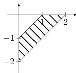
(a) La région V
