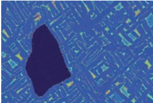
Sulfideinschluss im Eisenmeteorite Cape York. Dunkle Farbe zeigt die tiefe Nickelkonzentration im Sulfid (ca. 3 cm lang) in Vergleich zum umgebenden Metall (hellblau/grün).
