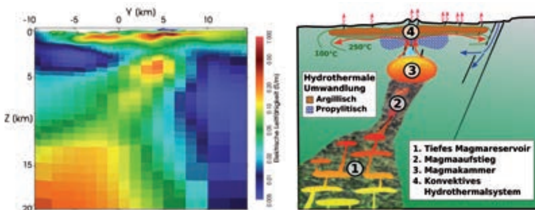
Untergrundmodell der elektrischen Leitfähigkeit eines Geothermalfelds im Ostafrikanischen Graben. Das Modell wurde durch 3D Inversion von magnetotellurischen Daten erzeugt und zeigt deutlich den typischen Aufbau eines vulkanischen Hochenthalpie Geothermie Systems. Die Studie entstammt einer Kollaboration zwischen der GEG Gruppe (Samrock, Saar), der EPM Gruppe (Grayver) und der isländischen Geothermiefirma Reykjavik Geothermal
