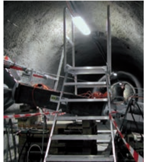
Plattendruckversuch im Felslabor Mont Terri.
