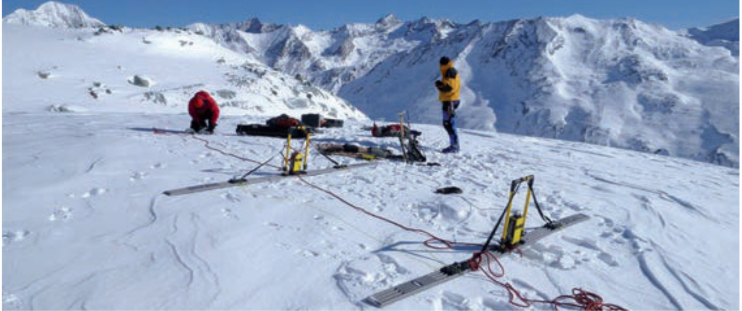
Bodenradarmessungen in den Schweizer Alpen.
