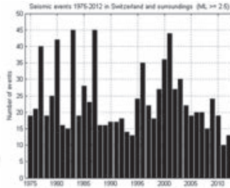
Erdbeben in der Schweiz von 1975 bis 2012 mit einer Magnitude von 2.5 oder mehr
