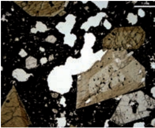
Mikroskopieaufnahme einer Lava, die Kristalle, Gasblasen und Glas (schwarz) enthält
