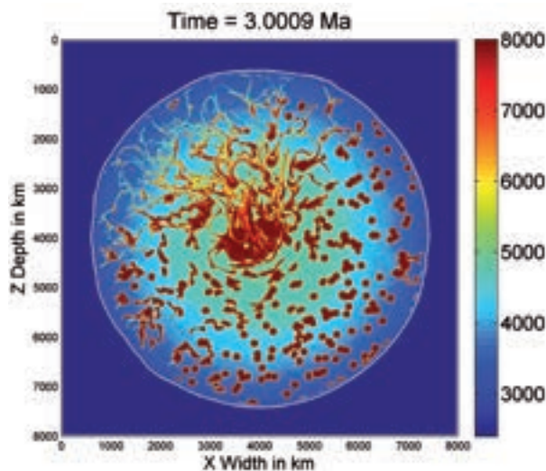
Computersimulation der Entstehung des Erdkerns durch absinkende Eisendiapire.
