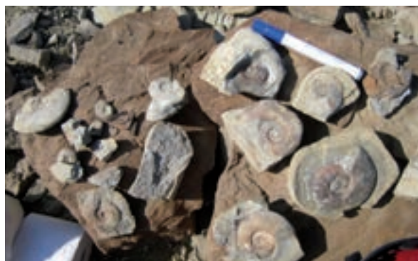
Basale Ophiceratid aus dem frühen Trias im Nordosten Grönlands.
