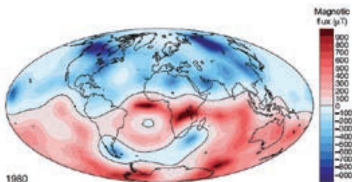
Darstellung des Erdmagnetfeld Flusses an der Oberfläche des Erdkerns im Jahr 1980
