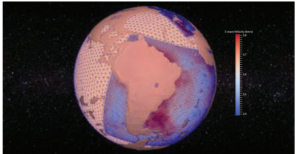
Modell der festen Erde bestehend aus Millionen kleiner Tetraeder, mit Topographie (überhöht) und Scherwellengeschwindigkeit in 100 Kilometer Tiefe.
