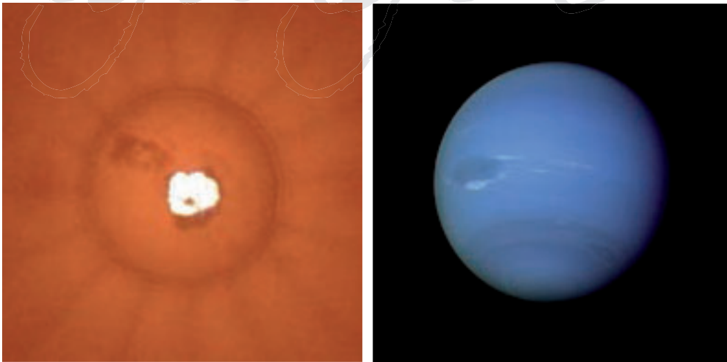
links: Mikroskopbild eine Probe in der Diamantstempelzelle bei einem Druck von 172 Gigapascal (1 72 Millionen mal atmosphärischer Druck). Der äussere Ring entspricht der Kalettenfläche des Diamantstempels und hat einen Durchmesser von 150 \mu\text{m} ; der innere Ring entspricht der Probenkammer und enthält Magnesiumsilikat als sogenannter \text{MgSiO}_3 Post Perovskit (Foto: Motohiko Murakami). rechts: Aufnahme des Neptun von der Voyager 1 Mission (Foto: NASA)
