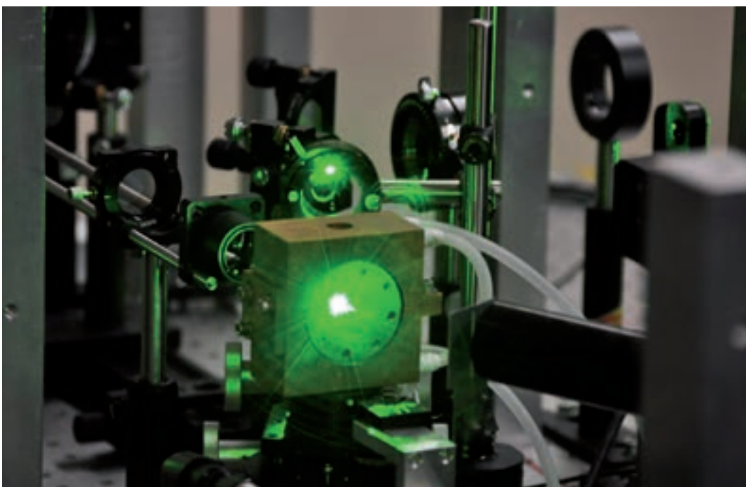
Diamantstempelzelle während einer spektroskopischen Messung (Foto John Hernlund).
