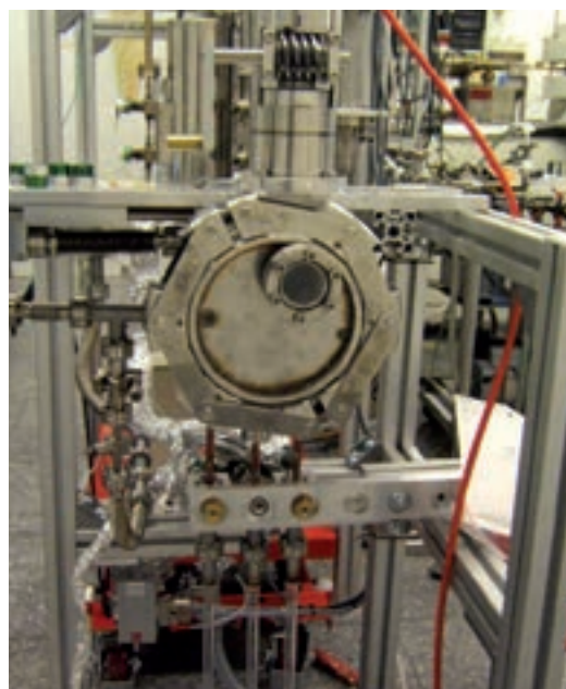
Eine selber entwickelte Mahl- und Siebmaschine, mit der die ursprüngliche Höhlentemperatur bestimmt werden kann: Sie misst die Konzentration von Edelgas im Wasser von Einschlüssen in den Stalagmiten.
