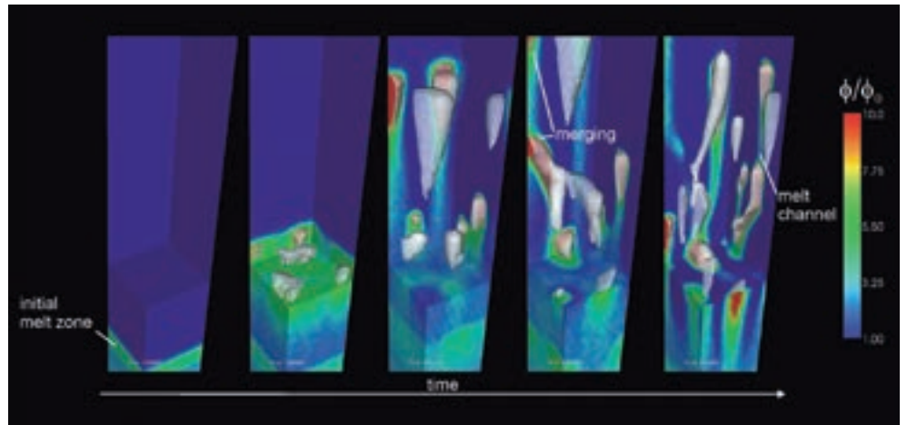
Numerische Simulation von Magmabewegung in partiell geschmolzenem Gestein.
