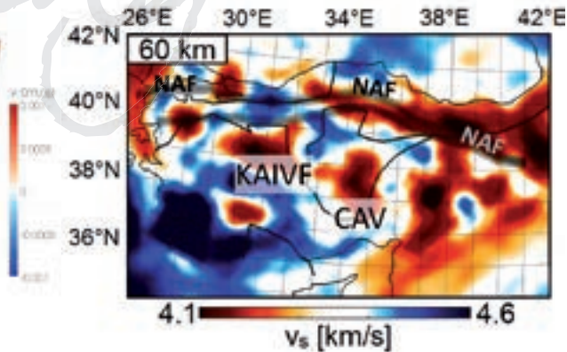
Scherwellengeschwindigkeit in 60 Kilometer Tiefe unter Anatolien. Gut sichtbar sind Niedriggeschwindigkeitszonen unter vulkanischen Provinzen (Kirka-Afyon-Isparta Vulkanfeld [KAIVF], Zentral-Anatolisches Vulkanfeld [CAV]) sowie die Signatur der Nordanatolischen Bruchzone (NAF), entlang derer sich regelmäßige große Erdbeben ereignen.
