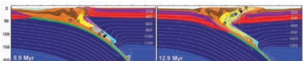
Numerische Modellierung der Kollision zweier tektonischer Platten.
