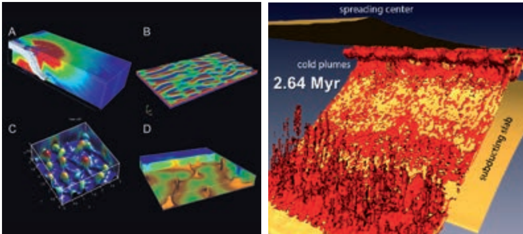
Computersimulation von verschiedenen geodynamischen Prozessen. A) Subduktion B) Gebirgsfaltung, C) Salztektunik D) Konvektion.
