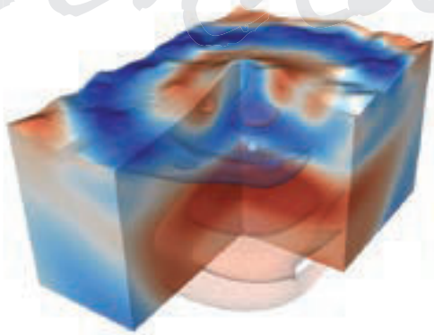
Ausbreitung seismischer Wellen durch ein Modell des Mount St. Helens.
