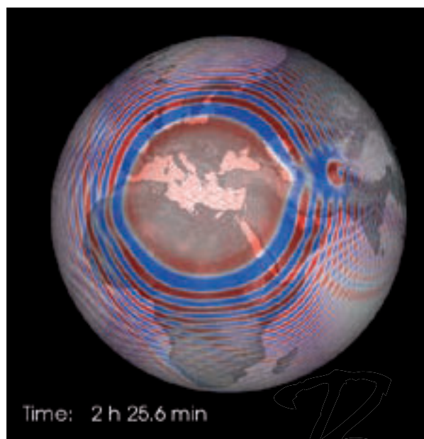
Simuliertes Erdbeben bei Kreta: Die Ausbreitung der Erdbebenwellen über den Globus.
