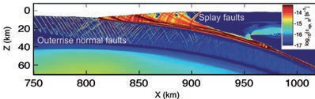
Numerisches Modell einer Subduktionszone, entlang welcher eine tektonische Platte (von links kommend) unter einen Kontinent (rechts) abtaucht. Rötliche Regionen repräsentieren Bruchzonen, die für hohe Erdbebenaktivität verantwortlich sind.
