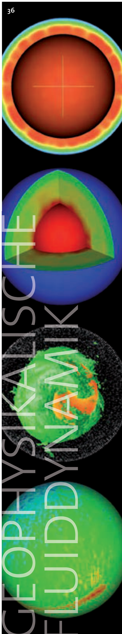
Numerische Simulation von Magmabewegung in partiell geschmolzenem Gestein.
