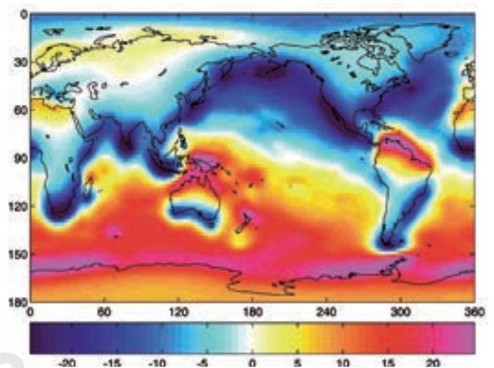
Der geomagnetische Sturm vom 5. 6. November 2001, dargestellt mit einem dreidimensionalen Modell, das auch die Flussdichte im Meer berücksichtigt.
