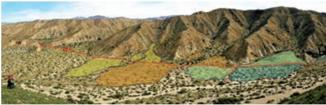
Versetzte geomorphe Merkmale entlang der San-Andreas-Verwerfung in Südkalifornien
