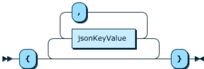
Figure 12.17 jsonDoc
