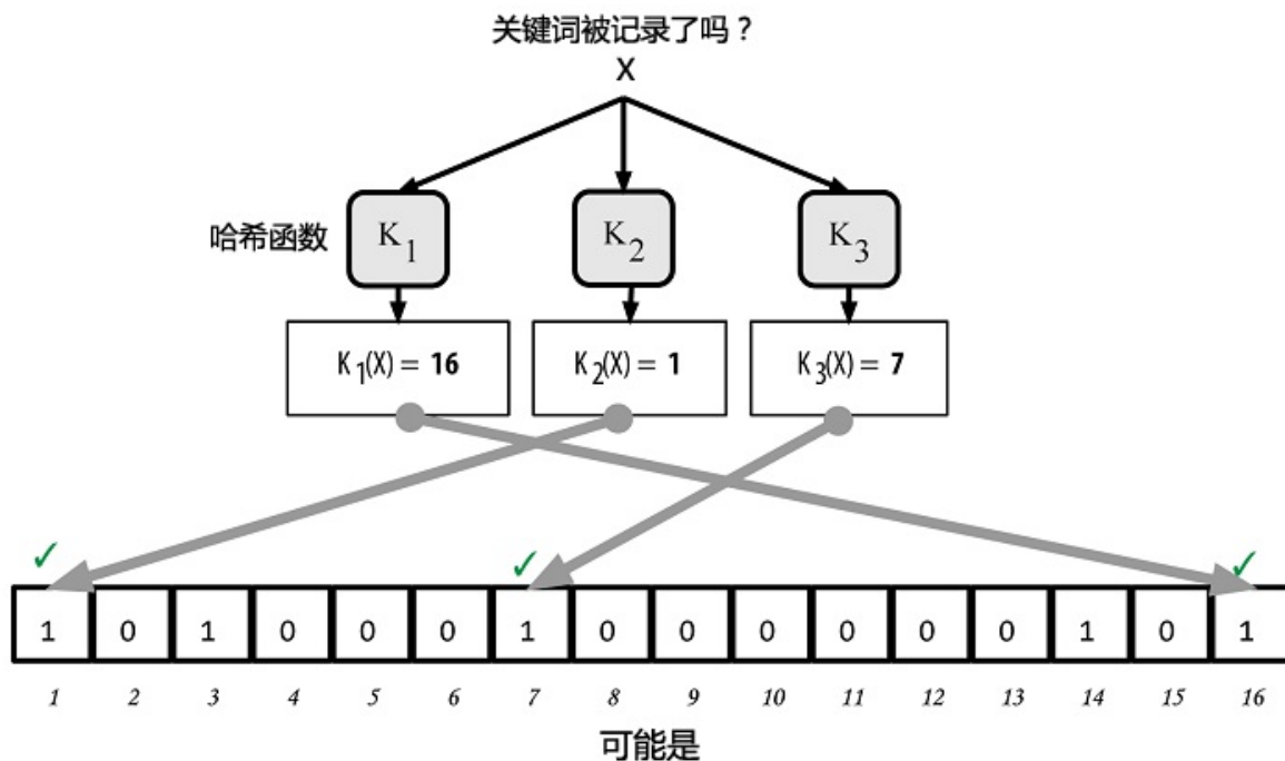
图6-11 验证关键词“X”是否存在于Bloom过滤器中。若结果为或然正匹配，则表示“可能是”。
