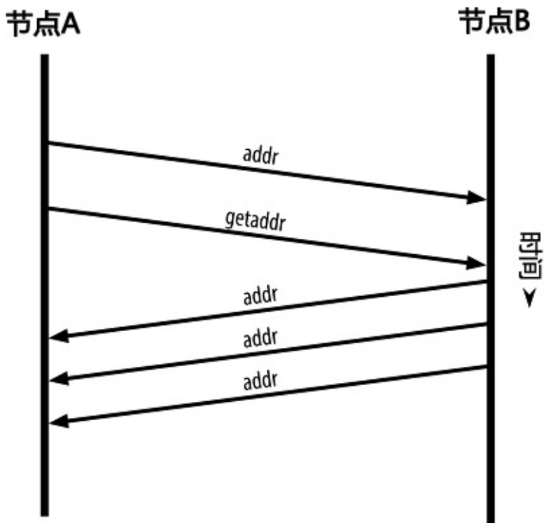
图6-5 地址广播及发现
