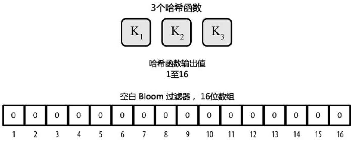
图6-8 一个由16位数组和三个哈希函数组成的简易Bloom过滤
