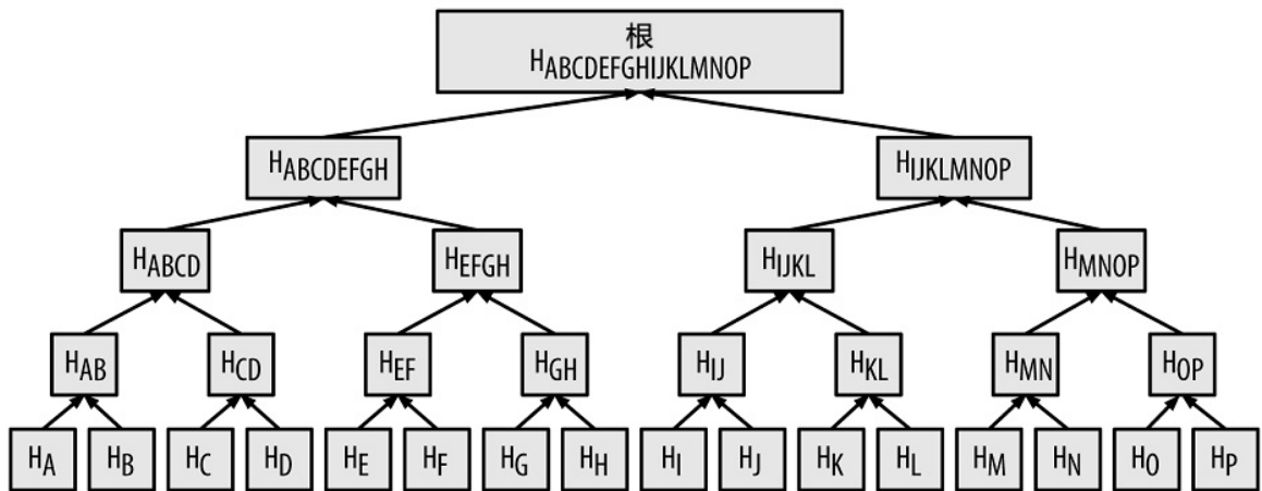
图7-4 一颗囊括了许多数据元素的Merkle树
