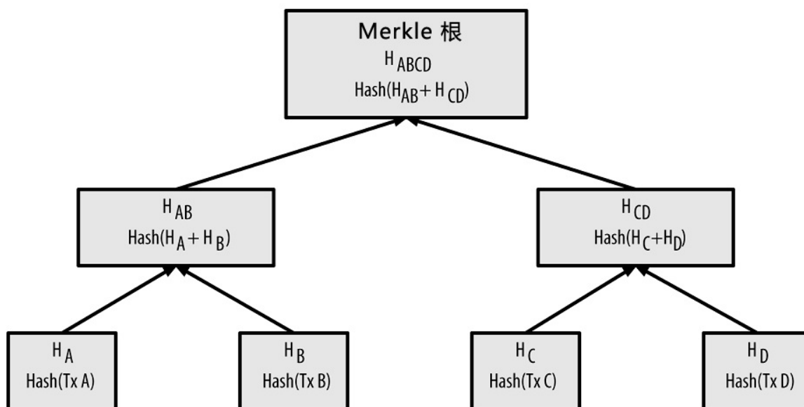
图7-2 在Merkle树中计算节点
