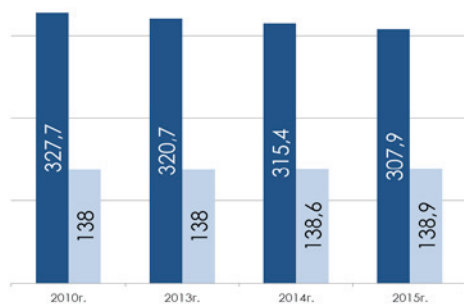
Рис. 4. Удельный расход топливно-энергетических ресурсов на производство электрической и тепловой энергии
